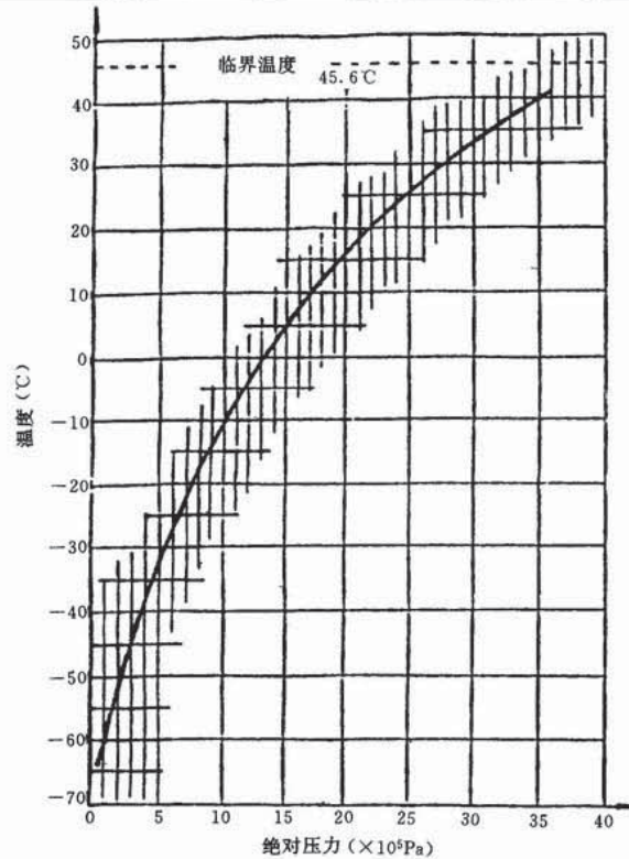
图1 六氟化硫的饱和蒸汽压曲线
